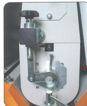
• Abjuster for rolling up or down 前砂輪高低調整
