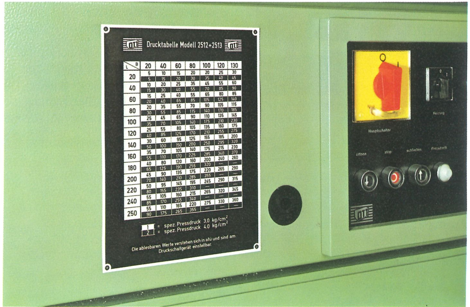
Drucktabelle mit 2 Wertangaben für Voll- und Teilbelegung der Preßfläche
