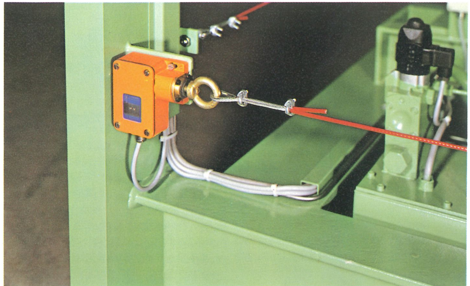
Sicherheits-Reißlinie über alle 4 Seiten der Presse.
