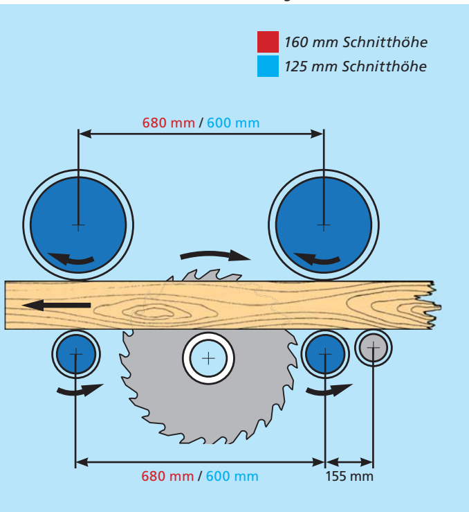
Abb. 11: Vorschubwalzenanordnung
