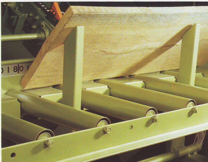
Aushebeeinrichtung für das Einsehen der Unterseite.
