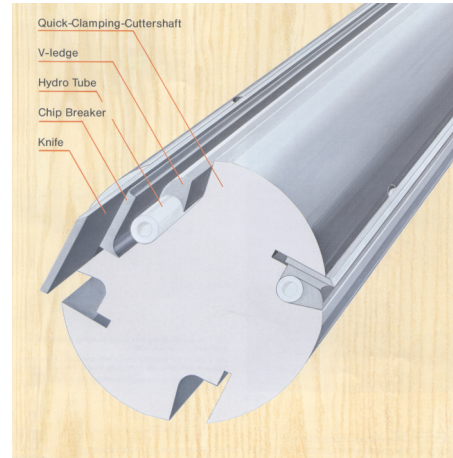
REX - Hydromesserwellensystem
