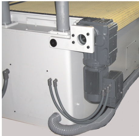
Transportband Vorschubsystem
