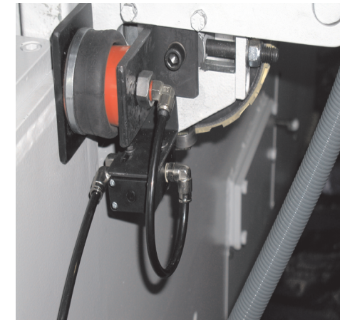
Pneumatische Bandzentrierung
