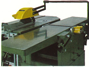
Kreissägeschutz- Vorrichtung
