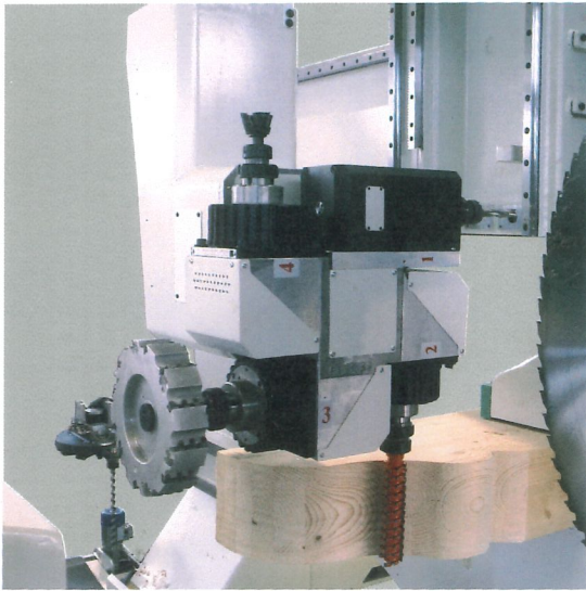
Unità operatrice a 5 assi controllati 4-star 5-axis head unit 4-Star
