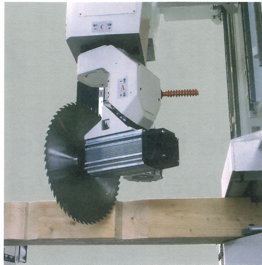
Unità di taglio lama a 5 assi 5-axis trimming unit with blade
