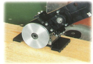
Querrippen-Schleppschuh von Schmidler. Patentiert!
