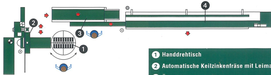
Vollautomat SK 20
