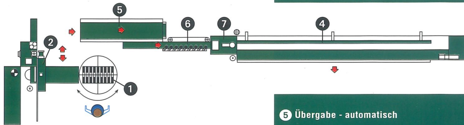
Vollautomat SK 20
