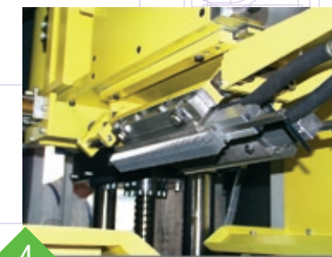
Klebstoffauftrag mit schwenkbarem Leimkammsystem Glue application with swiveling comb system
