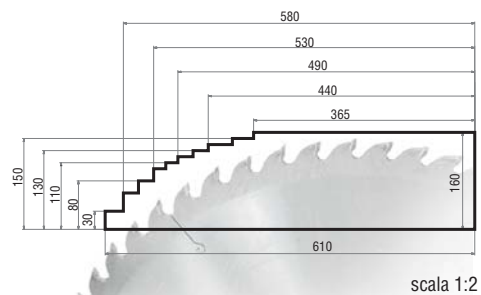
TR600 - Hp 12,5
