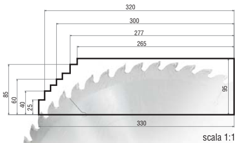
TR450 - Hp 5,5
