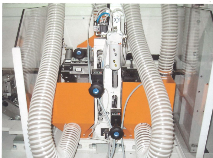
Gruppo finitore per alluminio Finishing unit for aluminium edge Grupo de retoque para aluminio
