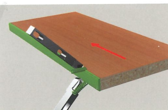
Gruppo raschiabordo Edgescraping unit Grupo rascador
