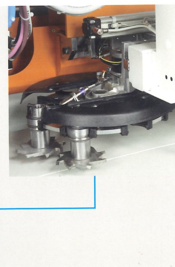
Gruppo raschiabordo multifunzione Multifunctional edgescraping unit Grupo rascador multifuncion
