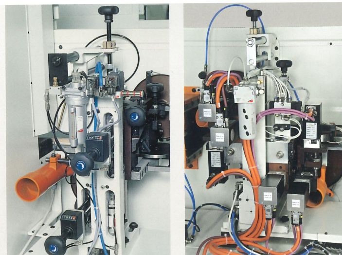
Gruppo raschiabordo multifunzione Multifunctional edgescraping unit Grupo rascador multifuncion
