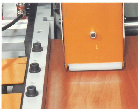
Dispositivo distanziatore pannelli Panel spacing device Dispositivo distanciador de paneles
