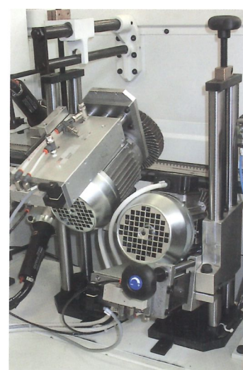
Gruppo spazzole per alluminio Buffing unit for aluminium edge Grupo cepillos para aluminio
