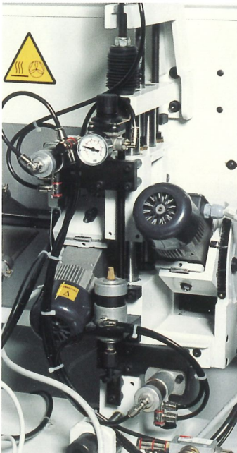
Gruppo tinteggiatore Staining unit Grupo coloreador
