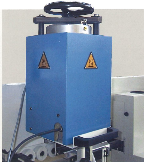
Kit applicazione colla poliuretànica (PUR) PUR glue process device Kit aplicaciòn cola poliuretànica (PUR)
