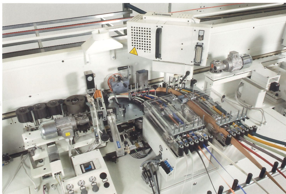
Gruppo incollaggio Gluing unit Grupo encolador
