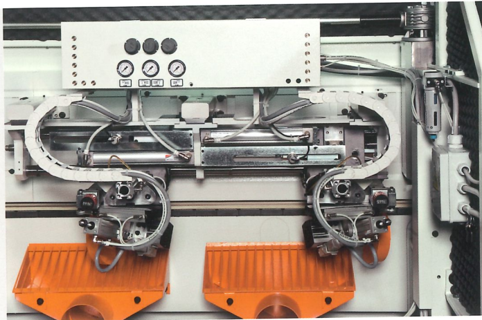
Gruppo intestatore End-trimming unit Grupo retesteador
