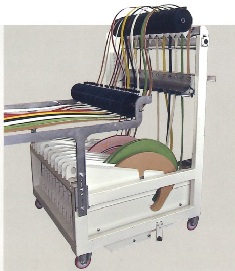
Portarotoli da 2 a 12 rotoli 2 to 12 coils holders Llevarollos desde 2 hasta 12 rollos
