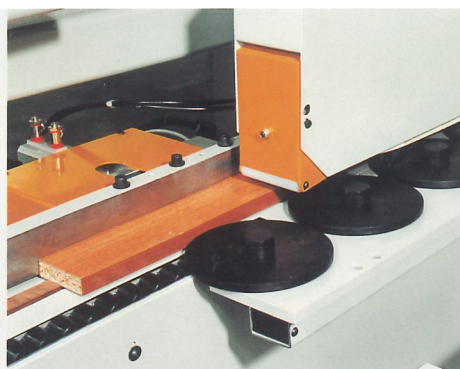
Barra a dischi per la lavorazione di pezzi stretti Disk-type counter pressure bar for processing narrow pieces Barra de discos para el trabajo de piezas estrechas
