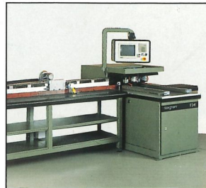
Fenster- und Türen-Bohrautomat FD-E Window and door dowel drilling ma- chine FD-E · Venster en deuren deuvell- boorautomaat FD-E
