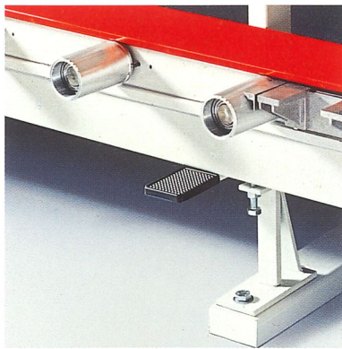
Gebremste Auflagerollen – sicherer Schutz vor unbeabsichtigtem Verschieben der Platten
