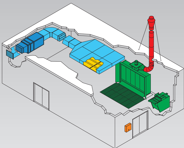
Schéma znázorňující energeticky úspornou vodní stěnu. Centrální stropní panel přívodu vzduchu vč. filtru.
