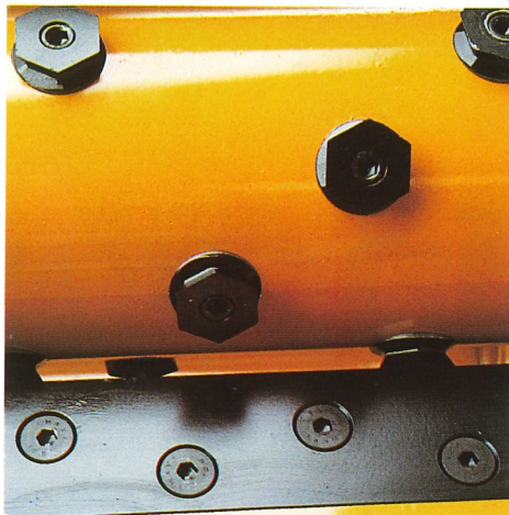
Rotor Langsamläufer mit mehrfach verwendbaren Schneidmessern.
