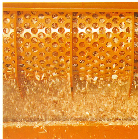
Lochsieb aus verschleißfestem Werkzeugstahl mit Verstärkungsrippen.
