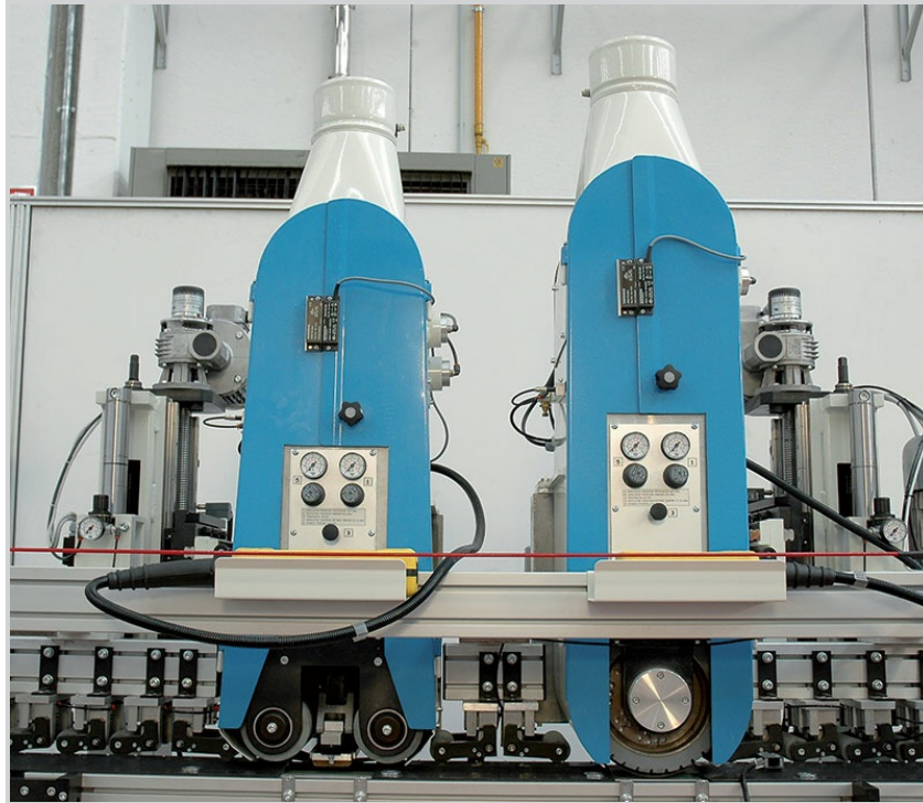
Breite Palette an Betriebseinheiten, Bänderinheit mit Rolle, Bänderinheit mit Puffer.
