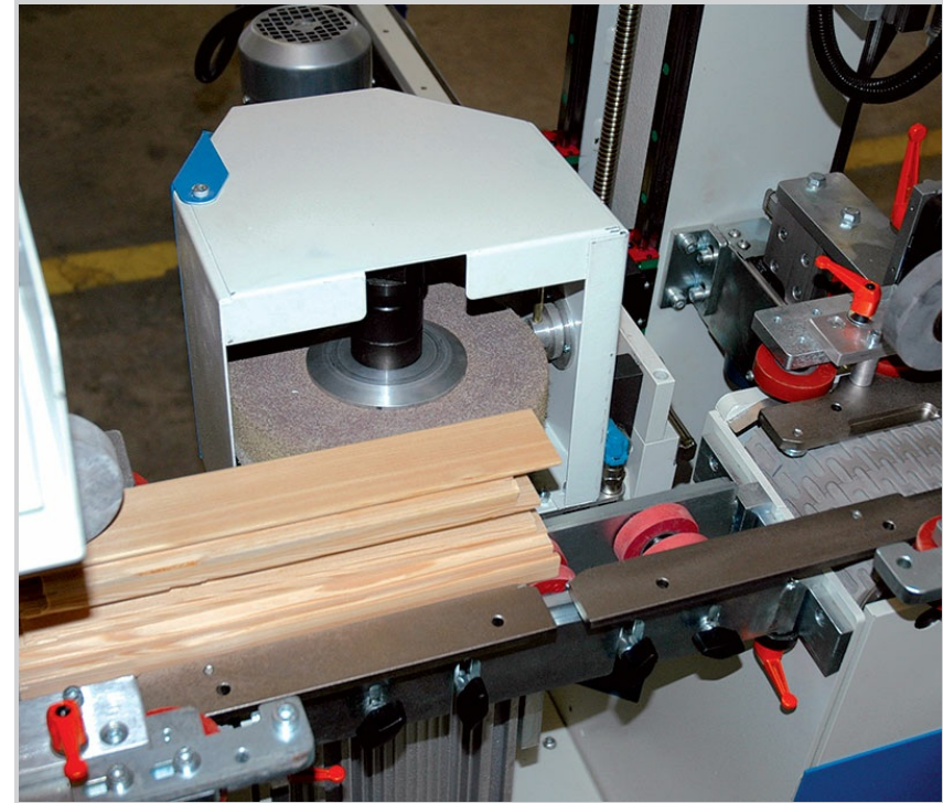
Schleifeinheit mit variabler Drehzahl, mit fester Schleifscheibe oder gezackter Schleifscheibe
