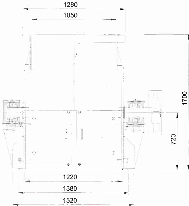
Frontansicht · front view · vue de face
