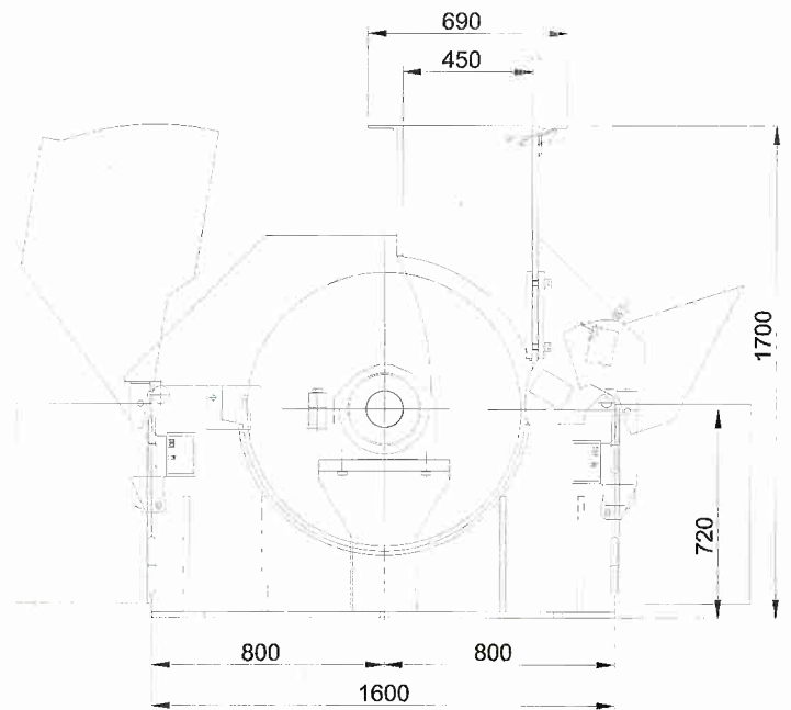
Seitenansicht · side view · vue de coté
