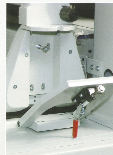
Robuste Tragbalkenverriegelung mit Einhandbedienung
