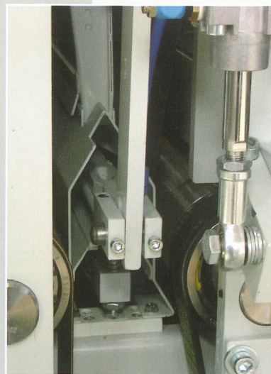
Schleifbandausblasung
