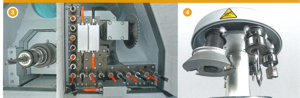
■ 18 Bohrspindeln vertikal ■ 6 Bohrspindeln horizontal ■ 1 Fräsmotor mit 9 kW HSK F 63 ■ 1 Nutsäge Ø 125 mm (0 / 90°)
