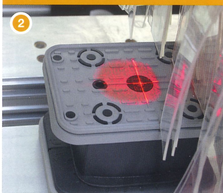
Einfaches Positionieren der Sauger durch den Fadenkreuzlaser
