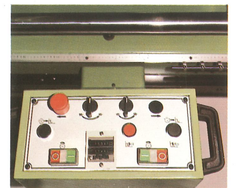
▷ Sicherheits-Zweihandsteuerung
