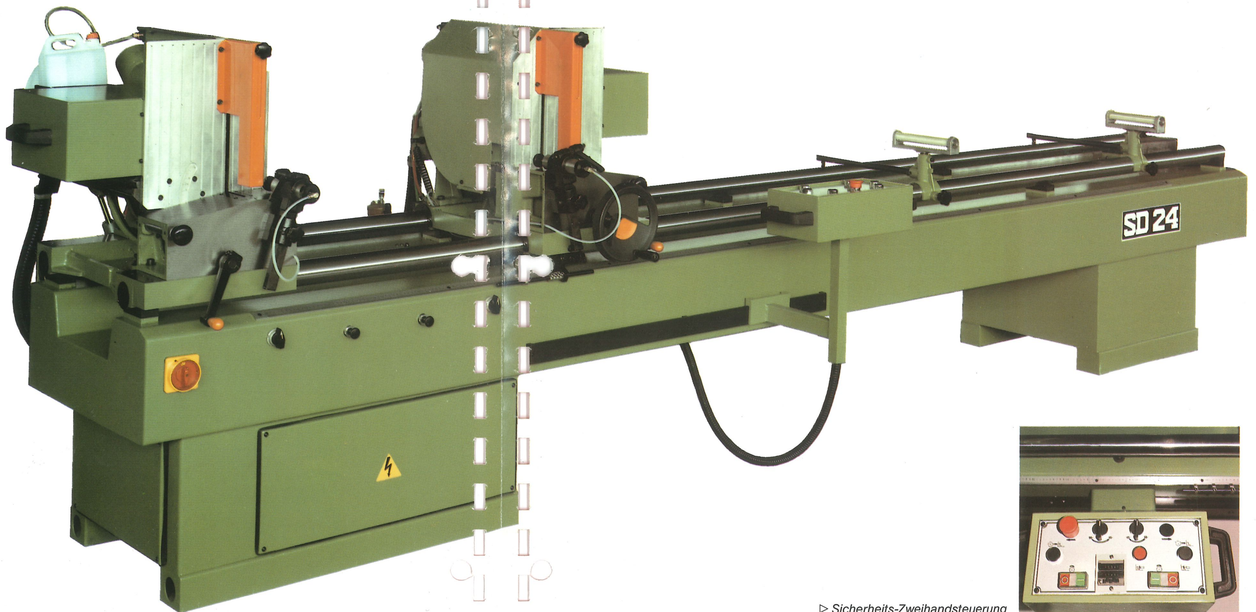
▷ Sicherheits-Zweihandsteuerung
