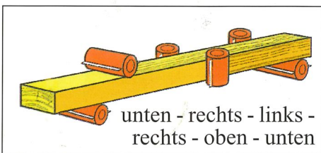
Die Spindelanordnung des Unimat 23 E Millennium
