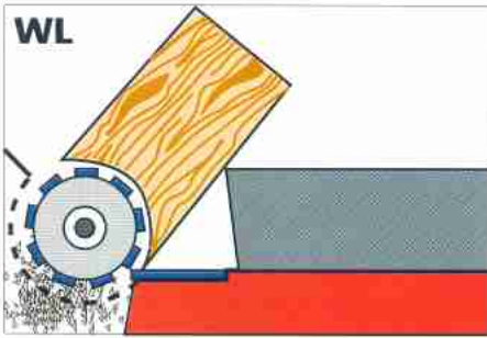
Rotor-Ø 368 mm
