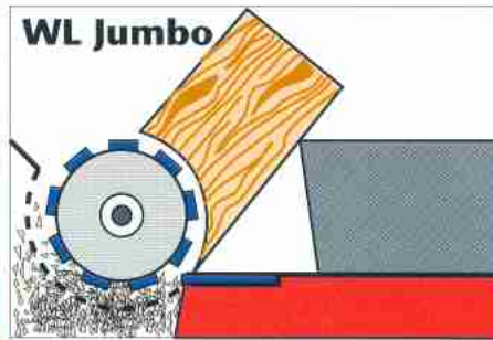
Rotor-Ø 482 mm
