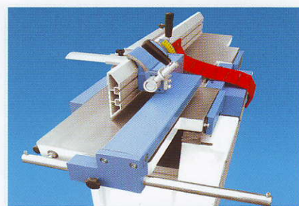
Професионален страничен линеал (DMA 41) Profi Seitenabrichtanschlag (DMA 41) Professional side fence (DMA 41)
