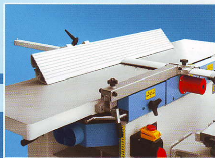
Наклон на линеала от 90° до 45° Abrichtanschlag von 90° auf 45° schwenkbar Fence tilting from 90° to 45°
