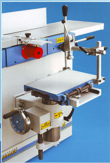
Борнапарат Langlochbohrereinrichtung Mortiser
