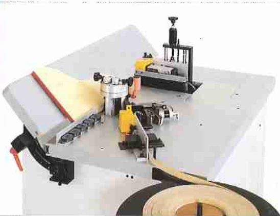
Possibilité d'incliner la table de travail.
