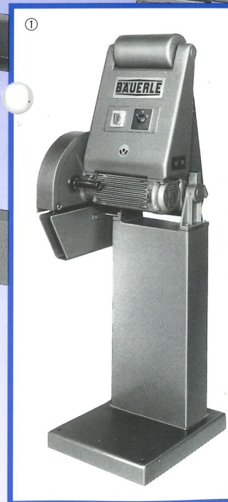
PKS mit starrem Ständer. Besonders stabil und preisgünstig. Höhe bis Mitte Sägeblatt h = 1050 mm Bestell-Nr. 33363
