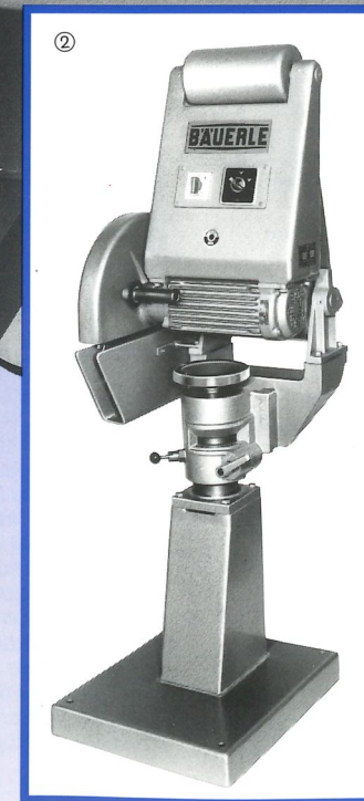
PKS mit Universalständer. Höhenverstg. um 75 mm zur vollen Ausnutzung des Sägeblattes und der Schnitthöhe. Höhe bis Mitte Sägeblatt h = 975 mm Bestell-Nr. 33365
