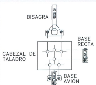
DETALLE CABEZAL 6 PORTABROCAS
