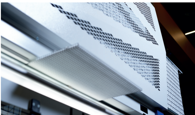
Alle Filter sind mit einem Schnellwechselsystem ausgestattet. 5 Filterebenen sorgen für optimale Umgebungsluft in der Lackierkabine.
