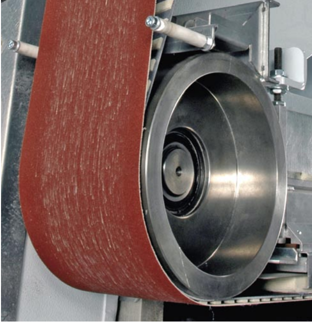
Die Querschleif-Einheit mit Elektronik-Schleifschuh
