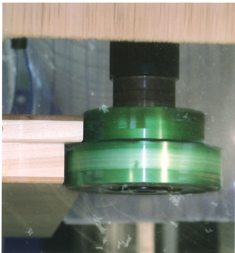
lavorazioni di porte da interni machining interior doors trabajos de puertas de interiores
