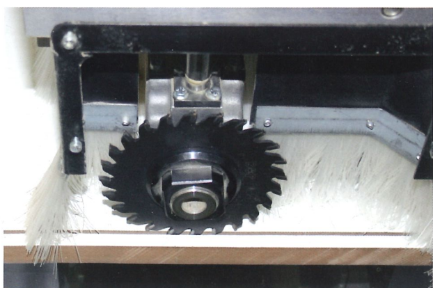
lavorazioni di componenti del mobile machining furniture parts trabajos de componentes del mueble
