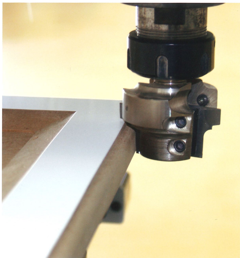
lavorazioni di componenti del mobile machining furniture parts trabajos de componentes del mueble
