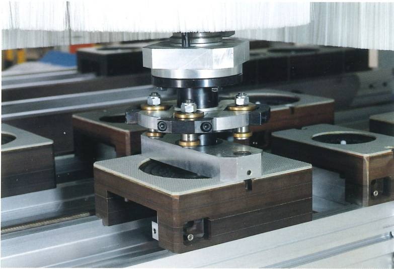
Positionnement automatique à CN des plans et des ventouses.
