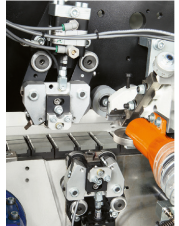
Flächenziehklingenaggregat „GS/K“ Beseitigung der Leimreste beim Plattenendbearbeitung
