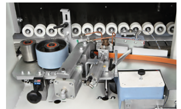
Anleimaggregat „GP 200“ Das Anleimaggregat ist mit zwei Andruckrollen und Kappschere für Kanten bis 3 mm Dicke aus- gerüstet. Das mit Teflon beschich- tete Leimbecken ist mit einem Schnellheizsystem und mit automatischer Vorrichtung für das Absenken der Leimtemperatur ausgestattet, welche die Zeiten zur Maschinenvorbereitung reduzieren.
