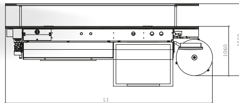
Kappaggregat „IK/200“ 2 Hochfrequenzmotoren, die sich von 0° - 15° einstellen lassen. Dadurch 2 Arbeitsmöglichkeiten möglich: Gerader Schnitt und Schrägschnitt
