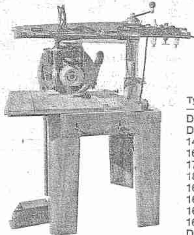
Typ 1600 mit aut. Vorschub und Tischverbreiterung vorn
