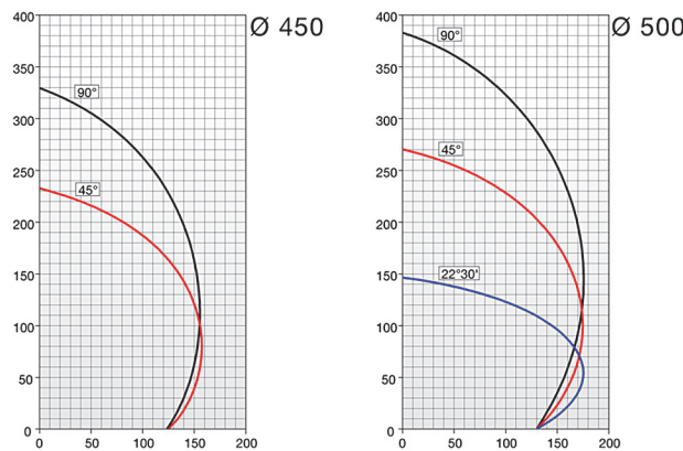
Schnittdiagramm
