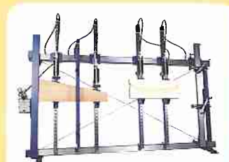
Schrägverleimung
