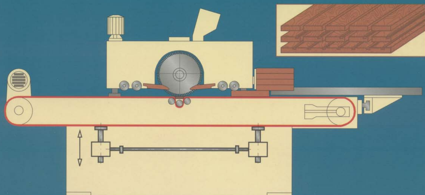
MESA DE ALTURA REGULABLE PARA RANURADO Y CORTE DE TABLEROS TABLE D'HAUTEUR RÉGLABLE POUR RAINURER ET COUPER DES PANNEAUX TABLE ADJUSTABLE IN HEIGHT FOR SLOTTING AND CUTTING BOARDS HÖHENVERSTELLBARER TISCH ZUM NUTEN UND SCHNEIDEN VON PLATTEN
