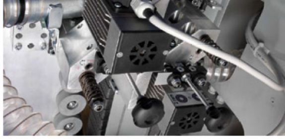
Gruppo regolatore multifunzione a regolazione veloce
