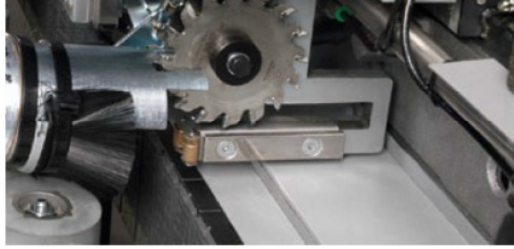
Gruppo motore ad alta frequenza e guide lineari di precisione
