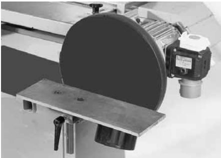
Tellerschleifeinrichtung mit abgedeckter Schleifscheibe.
