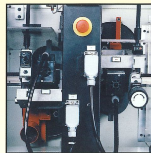
Spigolatore GS Top and bottom fine unit GS Espigador GS Fasenfräsaggregat GS Groupe à chanfreiner GS
