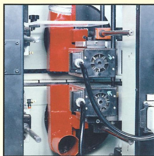
Refilatore GR Top and bottom rough unit GR Refilador GR Ebenfräsaggregat GR Groupe d'affleurage GR
