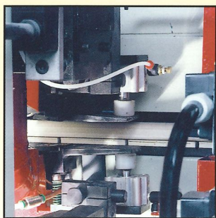
Raschiatore per soft GRF Scraping unit for soft GRF Rascador para sof GRF Ziehklingenaggregat GRF für Soft Groupe racleur pour soft GRF
