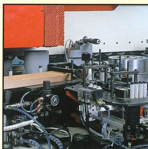
Gruppo incollaggio bordi dritti Unit for glueing straight edges Grupo de encolado para cantos rectos Aggregat zum Anleimen von geraden Kanten Groupe encollage chant droit
