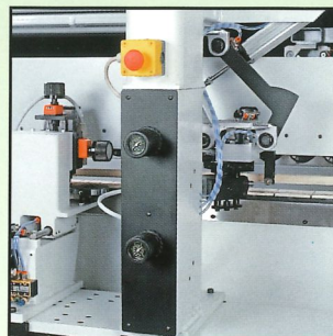
Gruppo fresatore bordo incollato bordatura trasversale Cope unit for processing of transversal edges Grupo fresador encolado, canteado transversal Fräsaggregat zur Bearbeitung der angeleimten Querante Groupe de fraiseage du bord transversal.
