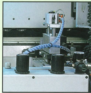
Scalpello pneumatico orizzontale Pneumatic horizontal chisel Zapata neumatica horizontal Pneumatisch gesteuerter Horizontal- Meißel Racleur pneumatique horizontal
