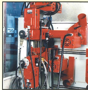
Incisore automatico inferiore 227K Incisore fisso superiore Bottom automatic scoring unit 227K Top fixed scoring unit Incisor automatico inferior 227K Incisor fijo superior Unteres autom. Vorritzaggregat 227K Oberes festes Vorritzaggregat Inciseur automatique inférieur 227K Inciseur fixe supérieur
