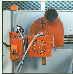
Truciolatore superiore inclinato Inclined top hogging unit Tritrador superior inclinado Oberes Zerspanaggregat mit Schrägstellung Déchiqueteur supérieur incliné
