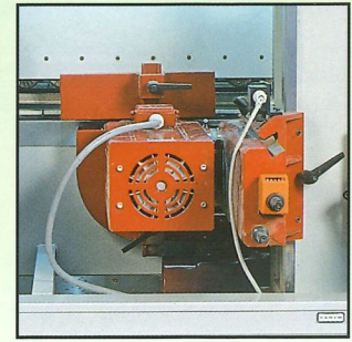
Truciolatore inferiore Bottom hogging unit Tritrador inferior Unteres Zerspanaggregat Déchiqueteur inférieur
