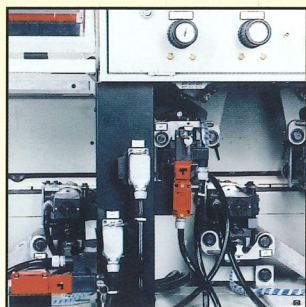
Copiatore / Arrotondatore G1-G2 Coping/corner rounding unit G1-G2 Copiador/redondeador G1-G2 Kopier-Abrundaggregat G1-G2 Groupe copieur/groupe à arrondir G1-G2
