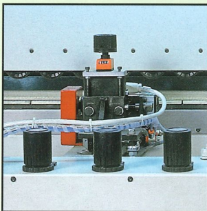
Intestatore bordo parte inclinata esterna End trimming unit for inclined outer side Retestador canto parte inclinada externa Kantenkappaggregat für schräge - Außenseite Coupe en bout de la partie inclinée extérieure
