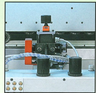
Intestatore bordo parte piana interna End trimming unit for flat inner side Retestador, canto parte recta interna Kantenkappaggregat für flache - Innenseite Coupe en bout du bord interieur
