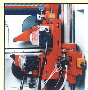
Profilatore orizzontale sup./inf. GPS Top/bottom horizontal profiling unit GPS Perfilador horizontal superior/inferior GPS Unteres u.oberes Horiz. Fräsaggregat GPS Groupe à profiler horizontal supérieur/inférieur GPS
