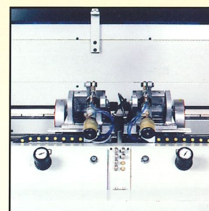
Intestatore GI End trimming unit GI Intestador GI Kappaggregat GI Groupe tronçonner GI
