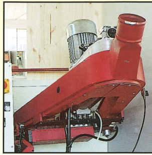
Levigatore a nastro per profili Belt sanding unit for profiles Lijador a banda para perfiles Profilbandschleifaggregat Groupe à poncer pour profils
