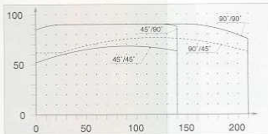
Schnittdiagramm GS 159/160 Cutting diagram GS 159/160 Diagramme de coupe GS 159/160 Geschwenkt / Gêneigt Turned / Tilted Orienté / Orienté et incliné
