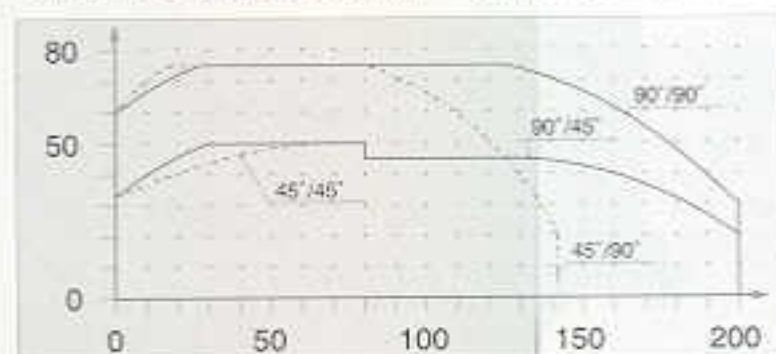
Schnittdiagramm GS 146/147 Cutting diagram GS 146/147 Diagramme de coupe GS 146/147 Geschwenkt / Gêneigt Turned / Tilted Orienté / Orienté et incliné
