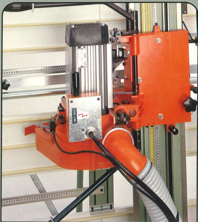
Sägeaggregat in horizontaler Stellung
