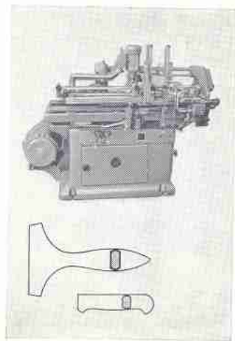
Kopierfräs-Automat Typ FP für Flachpinselstiele, Messergriffe und ähnliche Teile · Gleichzeitig mit 2 Fräsern nach Schablone arbeitend · Vollhydraulische Steuerung
