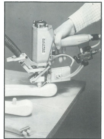
P12 mit verstärkter Schläufkraft für das Dübel-einschlagen in Hartholz
