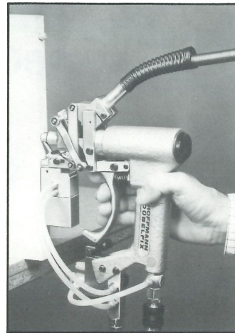
P11 für abgestapelte Werkstücke und Einzelwerkstücke (Innenausbau)
