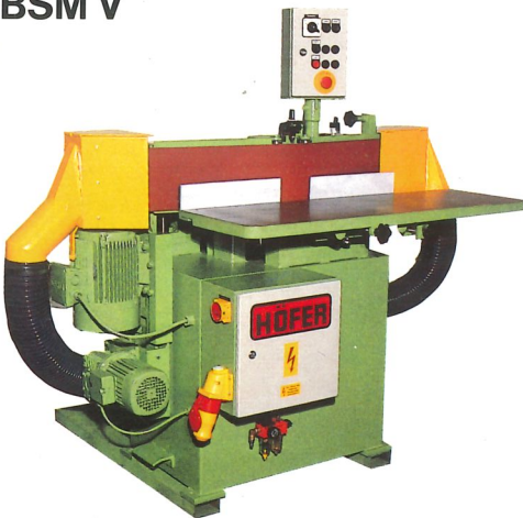
Doppelseitige Kantenschleifmaschine Two-side-edge sanding machine
