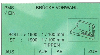
Druckbrückenhöhe
