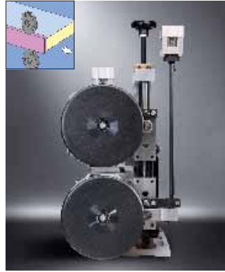
Rough trimming unit 0,55 or 1,5 kW
