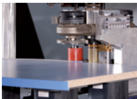
Placage de chants avec l'agrégat easyEdge
