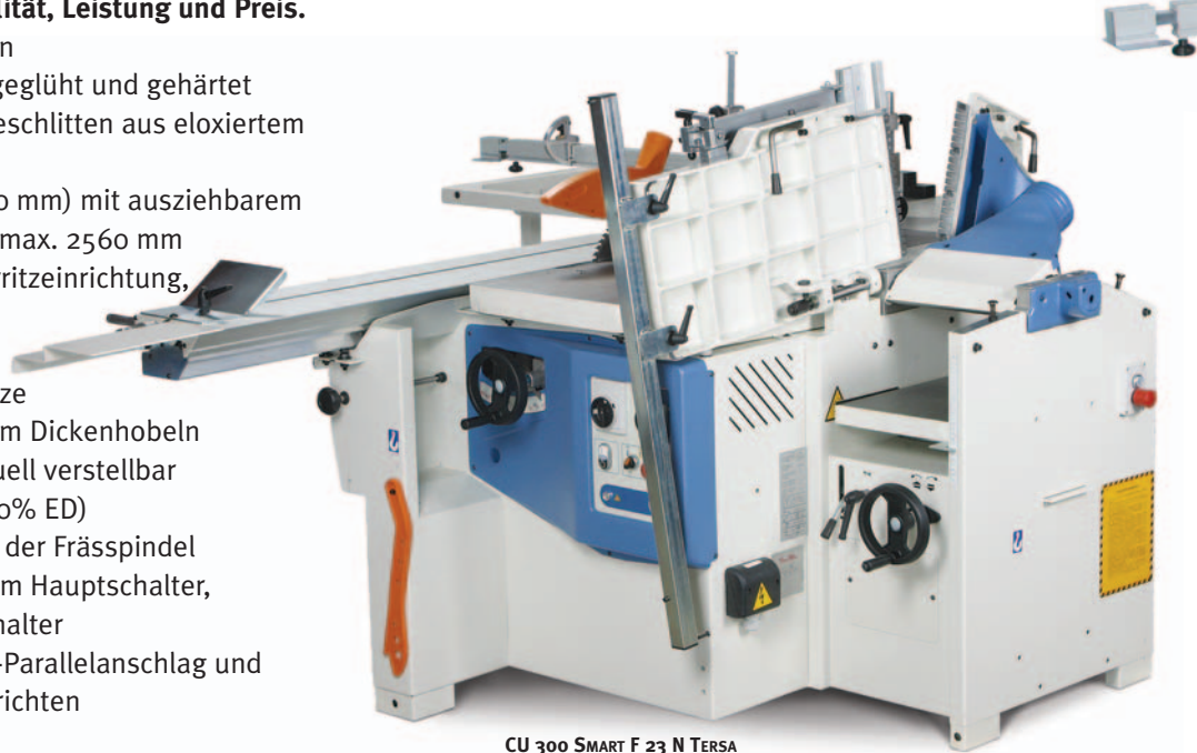
CU 300 SMART F 23 N TERSA mit nach innengeöffneten Abrichttischplatten
