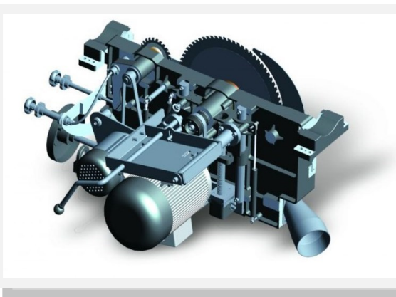
Sägeaggragat, max. Sägeblattdurchmesser 400 mm
