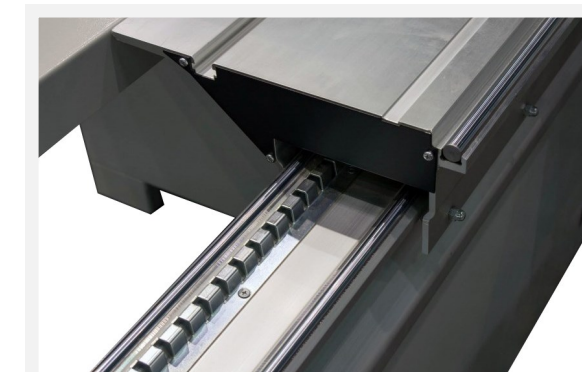
Schiebetischverriegelung stufenlos
