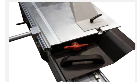
Groflachiger Tischausleger 1280 x 630 mm (verschiebbar) mit Materialrolle, Winkel- und Gehrungsanschlag (ausziehbar bis 3400 mm)
