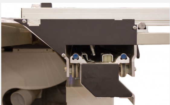
Stabiles Schiebetischprofil 420 mm mit praziser Rundstangenfuhrung, dauerhaft leichtgangig, Staub- und Schmutzunempfindlich
