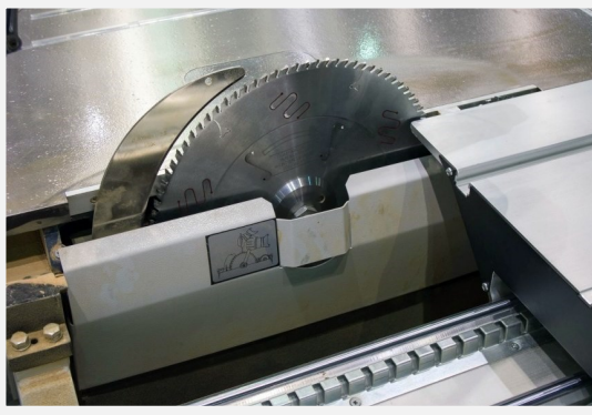
Sägeaggragat, max. Sägeblattdurchmesser 400 mm
